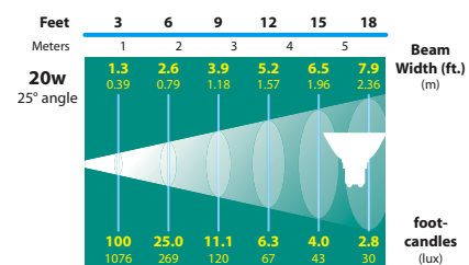
20w ALR12 FL (GBF) SL-34-ALR12
