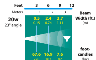
20w MR8 FL SL-34-MR8, SL-39
