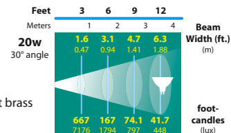
20w MR11 FL (FTD) SL-34-MR11
